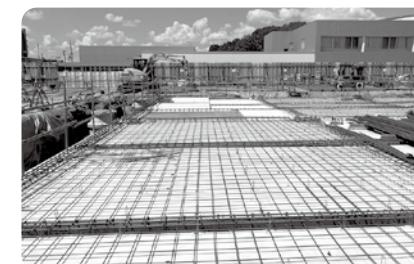
1Fスラブ型枠の施工状況 (2026.9.1 現在) スラブ型枠：床のコンクリート (スラブ) を流し込んで固めるための型枠のこと
